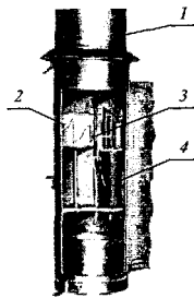
Рис. 7.4. Плювиограф П-2:
