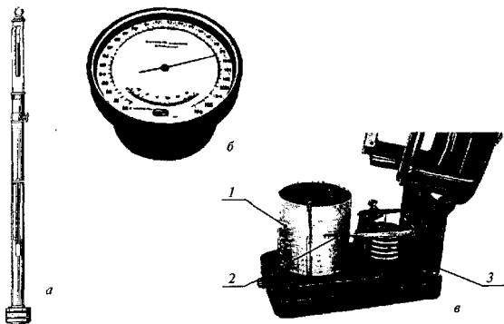
Рис. 1.1. Приборы для измерения атмосферного давления:
