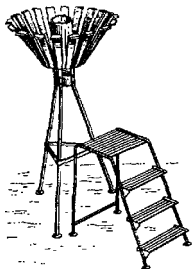
Рис. 7.2. Осадкомер Третьякова О-1
