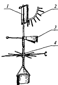
Рис. 9.3. Флюгер станционный (Вильда) ФВЛ, ФВТ:
