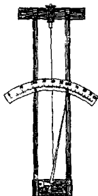
Рис. 5.6. Волосной гигрометр МВ-1
