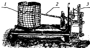
Рис. 5.7. Гигрограф волосной М-21А:
