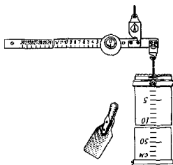
Рис. 7.5. Весовой снегомер ВС-43
