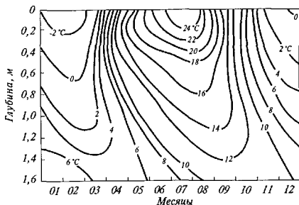
Рис. 3.5. Термозоплеты годового хода температуры почвы в районе (г. Харьков)
