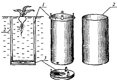
Рис. 6.1. Почвенный испаритель ГГИ-500-50:
