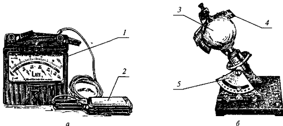
Рис. 2.6. Приборы для измерения освещенности (а) и продолжительности солнечного сияния (б):
