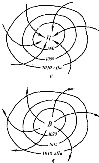
Рис. 9.7. Схемы барических систем:
