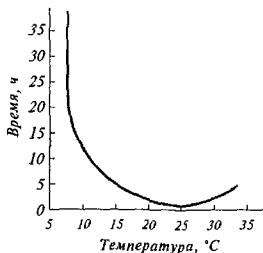
Рис. 4.8. Зависимость прорастания конидий возбудителя оидиума винограда от температуры воздуха (по Я. А. Сейдаметову, 1938)
