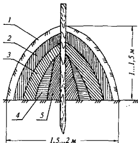
Рис. 12.10. Дымовая куча:
