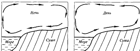
Рис. 9.9. Схема бризов
