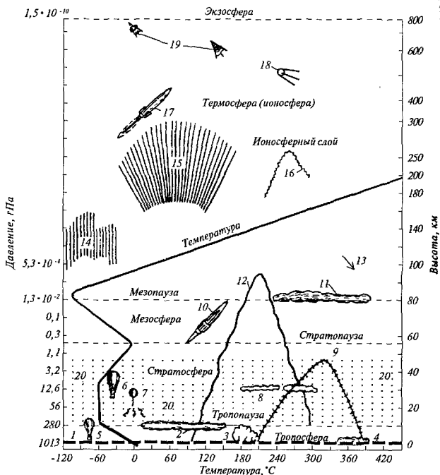
Рис. 1.2. Строение атмосферы:
