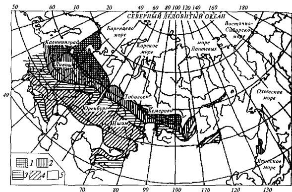
Рис. 8.3. Агрогидрологические зоны:
