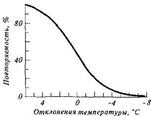
Рис. 11.8. Повторяемость отклонений годовых минимумов температуры от среднего из абсолютных годовых минимумов
