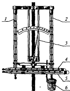
Рис. 5.4. Установка приборов в психометрической будке:
