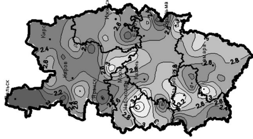
Рис. 5.2. Средняя скорость ветра (м/с) в январе (слева) и в июле (справа)
